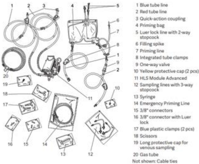
Figura 1: Línea de tubo azul (1), Línea de cebado de emergencia (14)
