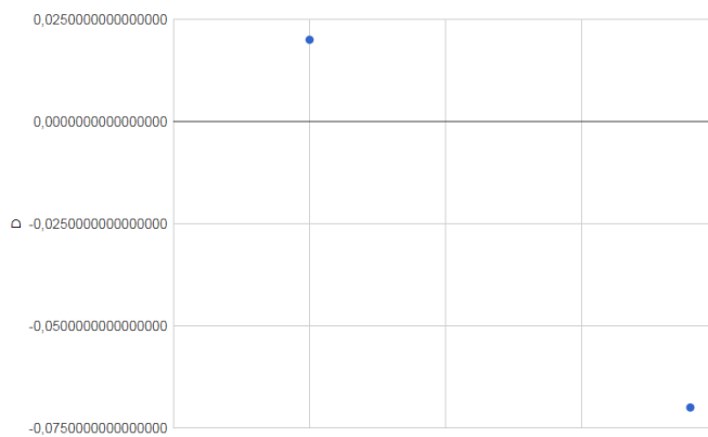
GRÁFICA N° 14. Dispersión de datos para determinación de 2,4 – Dinitrotolueno.
