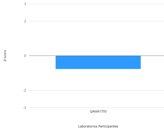
GRÁFICA N° 10. Distribución de z-score para determinación de 2,4 – Dinitrotolueno.
