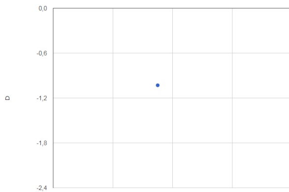
GRÁFICA N° 14. Dispersión de datos para determinación de 2,4 – Dinitrotolueno.
